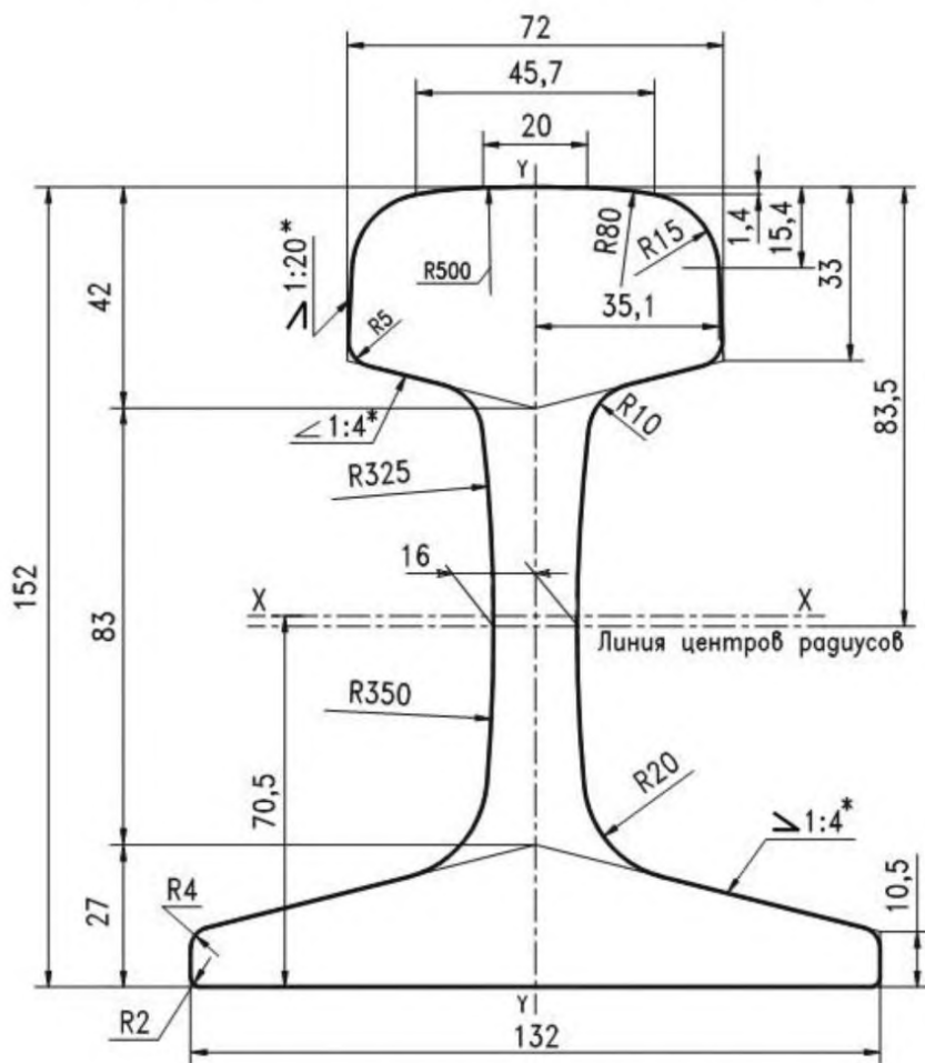
Рисунок А.1 – Рельс типа РГ50
