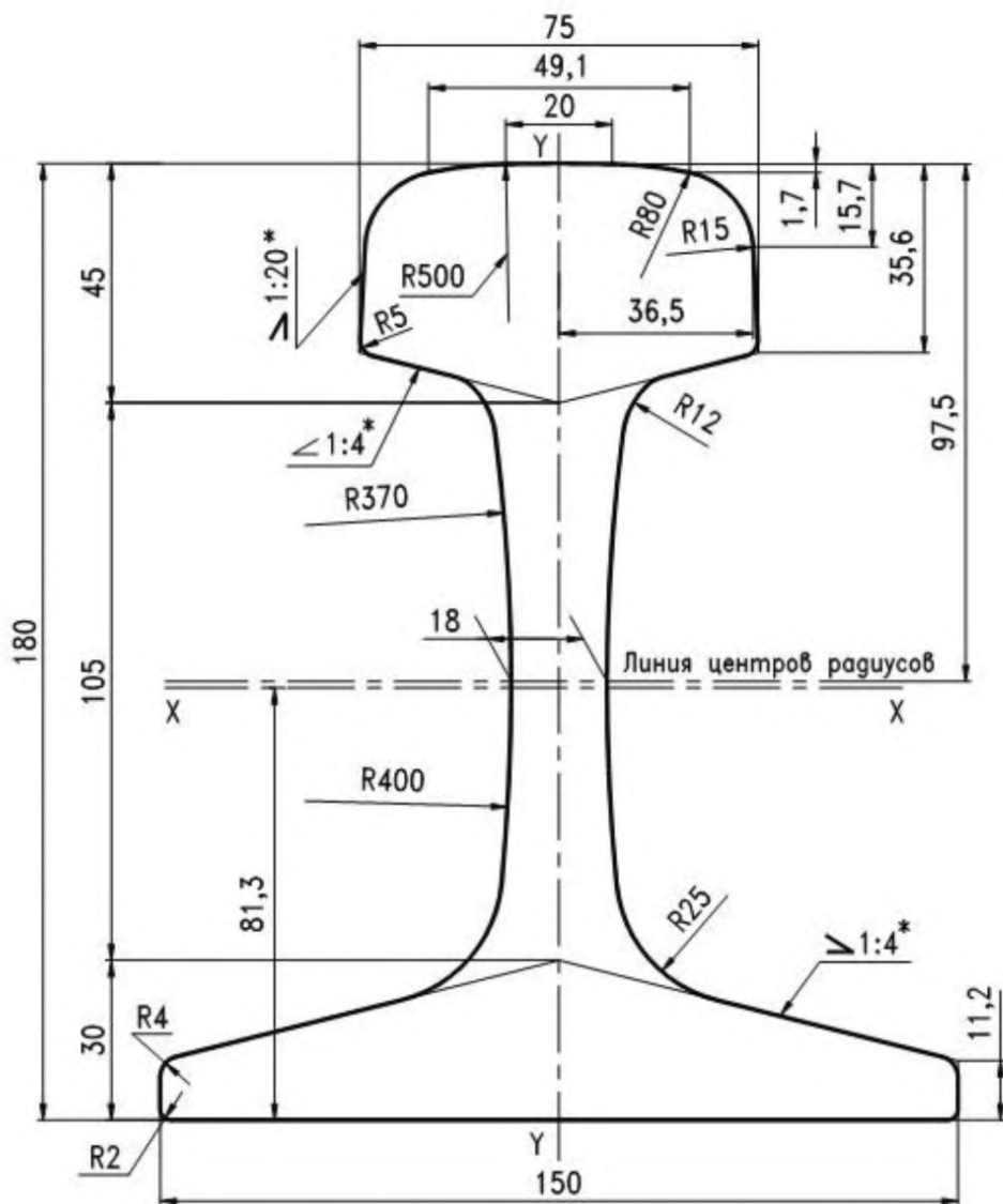
Рисунок А.3 – Рельс типа РП65
